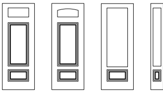
95" Door for 22 × 9" doorlite 95" Door for 22 × 9" camber top doorlite 95" Door for 22 × 64" doorlite 95" Sidelite for 7 × 64" lite
