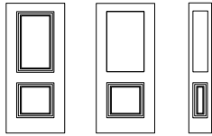
79" Door 79" Slab for 22 × 36" doorlite 79" Reversible Sidelite for 8 × 36" lite
